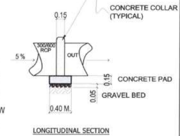
LONGITUDINAL SECTION
