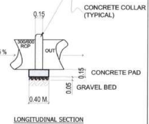
LONGITUDINAL SECTION
